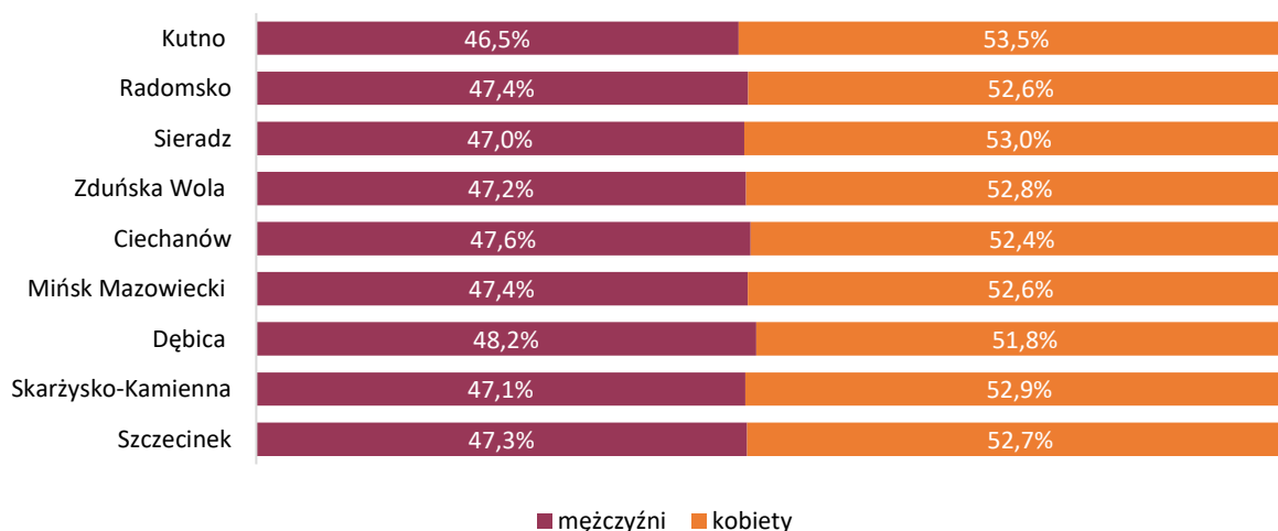
WYKRES 1. STRUKTURA LUDNOŚCI MIAST GRUPY PORÓWNAWCZEJ ZE WZGLĘDU NA PŁEĆ W 2022 ROKU
