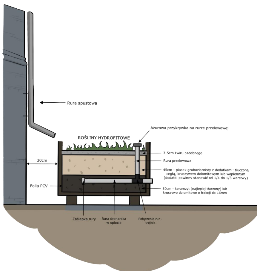
Rysunek 35 Schemat budowy ogrodu deszczowego w pojemniku (Opracowanie własne na podstawie opracowania Ogród deszczowy w pojemniku, Fundacja Sendzimira)
